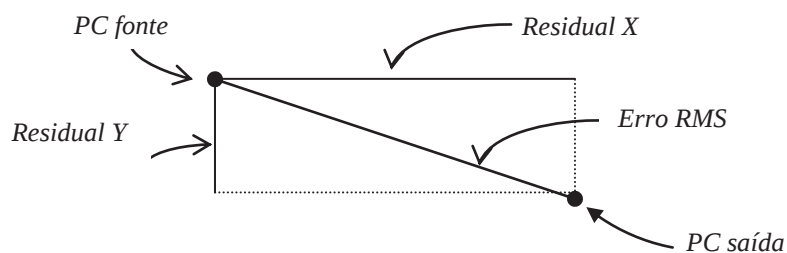
Fig. 6.14 Representação geométrica da medida do erro RMS de um ponto de controle.
