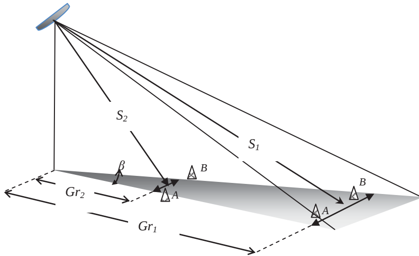
Fig. 4.10 Dependência da resolução azimutal em função das distâncias S medidas no plano inclinado, ou da abertura angular \beta do lóbulo de iluminação do feixe de radar.
