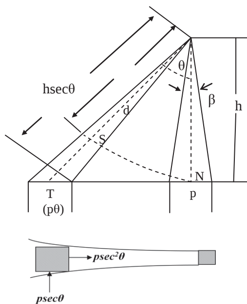
Fig. 6.9 Distorção geométrica da imagem devido à visada cônica, causando deslocamento e aumento da área do pixel.
