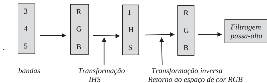
Fig. 8.9 Etapas do processo de transformação do espaço de cores RGB para o espaço IHS.
