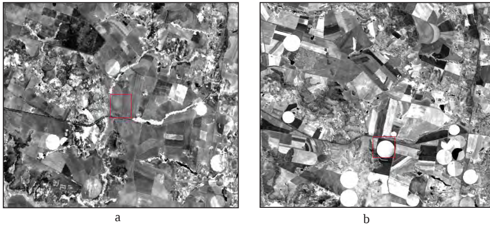
Fig. 1.25 Imagens Landsat de área agrícola obtidas nos anos de 2000 (a) e 2009 (b). Notar o crescimento de pivôs centrais e a modificação do parcelamento dos cultivares.
