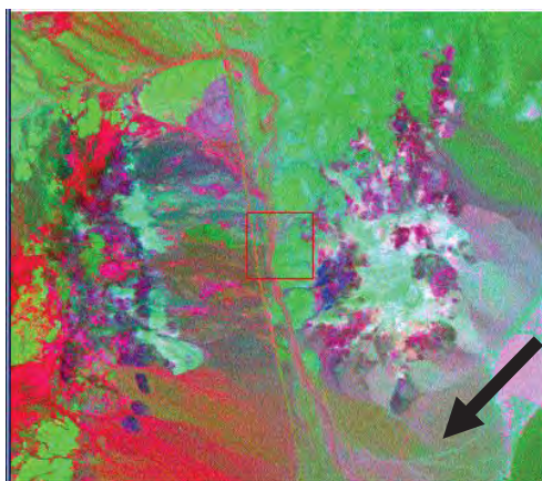
Fig. 14.21 Composição colorida com a imagem linear spectrum unmixing para os endmembers illita em vermelho, calcita em verde e RMS em azul.
