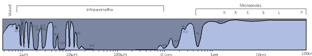
Fig. 1.9 Transmissância ( T ) da radiação eletromagnética através da atmosfera. As áreas em azul correspondem às regiões espectrais de transparências da atmosfera e as áreas em cinza correspondem às regiões espectrais onde os gases atmosféricos absorvem a radiação eletromagnética.
