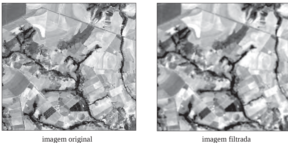
Fig. 11.7- Efeito de suavização da imagem por filtro passa-baixa de tamanho 5 \times 5 .
