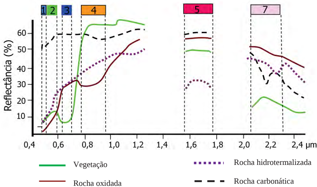
Fig. 8.6 Espectros de reflectância de quatro materiais e as posições das bandas do sensor ETM como meio prático para selecionar três bandas que melhor possam identificar esses materiais.
