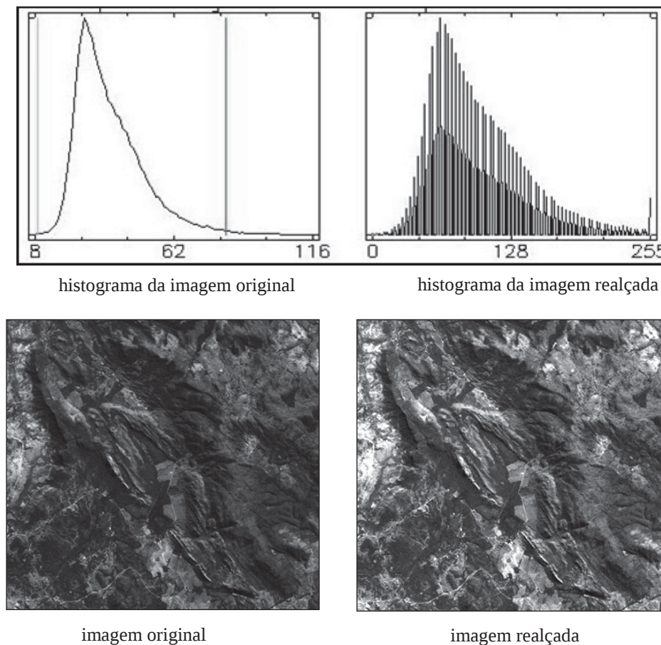
Fig. 7.6 Exemplo de realce de contraste por expansão linear histogrâmica de imagem ETM da banda 7 e respectivos histogramas da imagem original e modificada.
