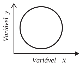
Fig. 10.9 O círculo representa o espaço de uma distribuição entre duas variáveis não correlacionadas.
