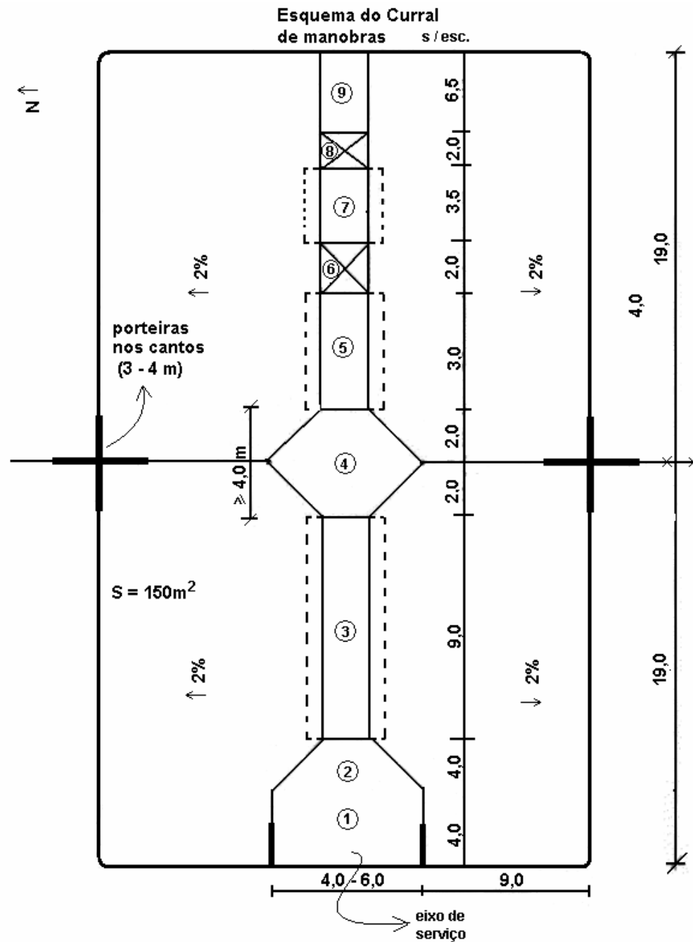
Croqui de curral de manobras dimensionado para 300 bois.
