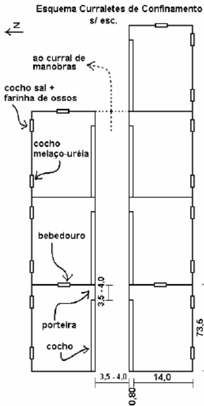
Figura 3 –Curral de Confinamento composto por sete curraletes.
